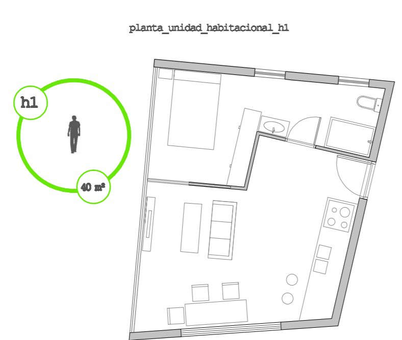
plantas unidades habitacionales h1 h2 h3 h4 h5 e 1:100
